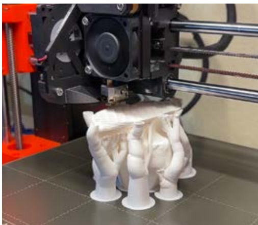
Ein neuer Kopf entsteht im 3D-Drucker mit Stützstrukturen, ...
